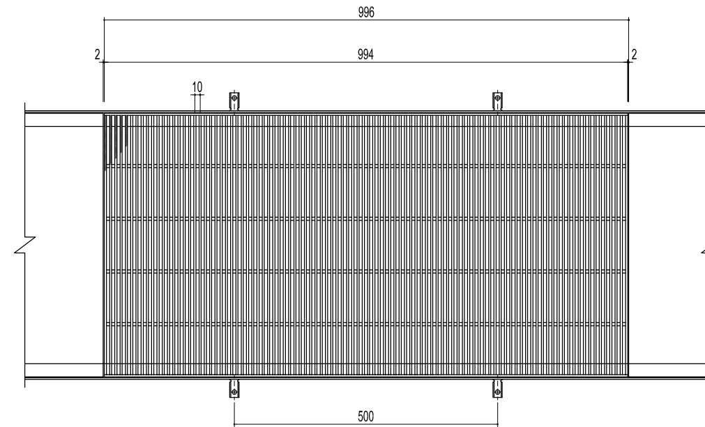
MẶT BẰNG CHI TIẾT
