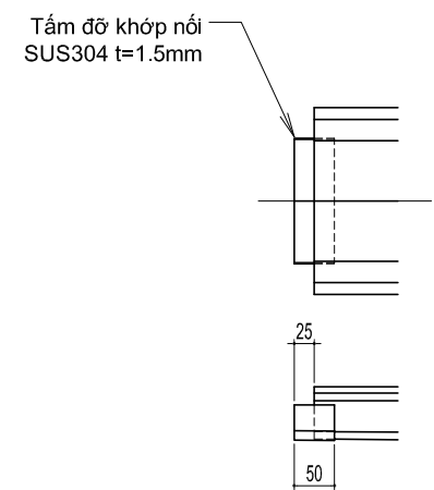
TẤM ĐỠ KHỚP NỐI SL: 1/5
