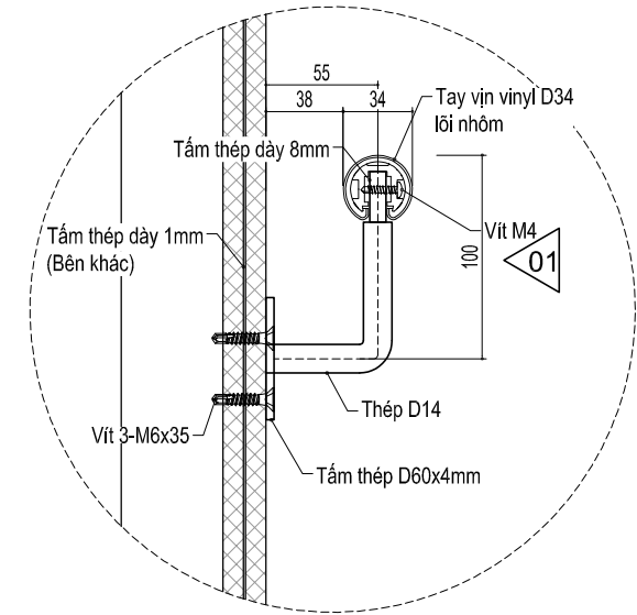
CHI TIẾT LOẠI A2 TAY VỊN CHO TƯỜNG THẠCH CAO
