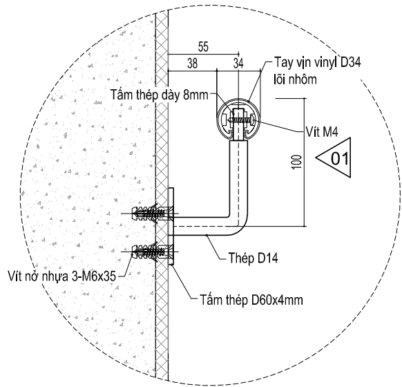
CHI TIẾT LOẠI A1 TAY VỊN CHO TƯỜNG BÊ TÔNG
