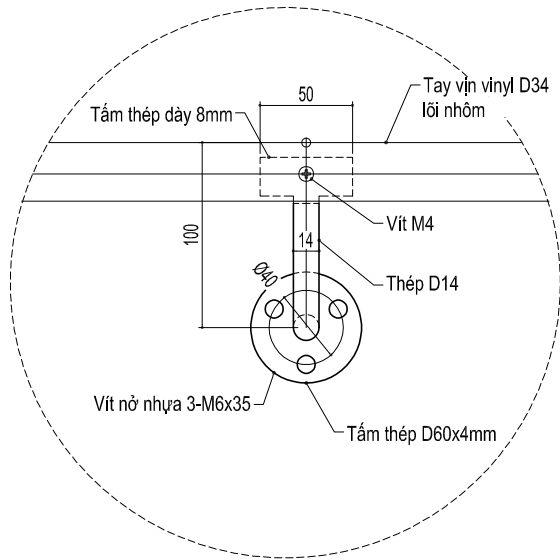
CHI TIẾT LOẠI A1 TAY VỊN CHO TƯỜNG BÊ TÔNG HƯỚNG NHÌN 1
