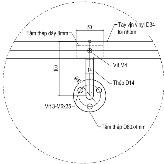
CHI TIẾT LOẠI A2 TAY VỊN CHO TƯỜNG THẠCH CAO HƯỚNG NHÌN 1
