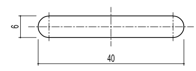
CHI TIẾT LỖ THOÁT NƯỚC SL: 1/2
