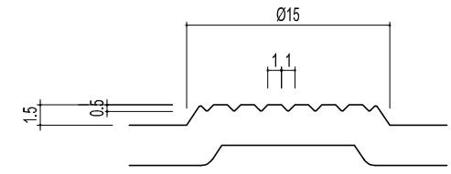
CHI TIẾT CHỐNG TRƯỢT SL: 1/4
