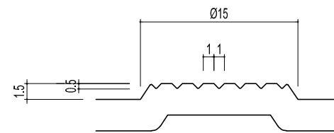
CHI TIẾT CHỐNG TRƯỢT SL: 1/4
