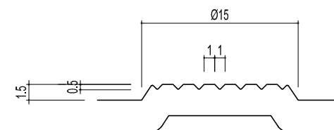
CHI TIẾT CHỐNG TRƯỢT SL: 1/4
