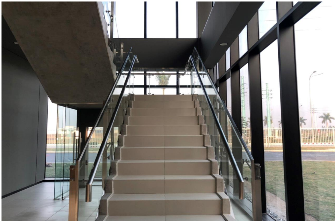
Hạng mục Lan can kính cầu thang – Dự án Nhà máy Yamamoto Việt Nam Category: Glass staircase railing – Yamamoto Vietnam Factory Project
